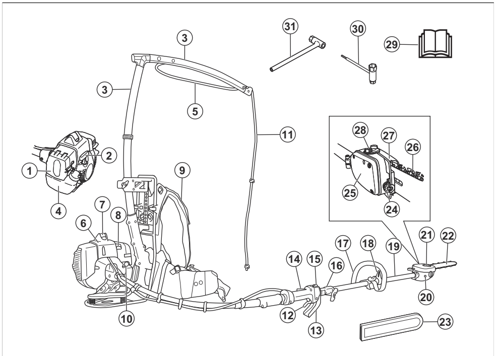
1. Luftfilterdeckel
